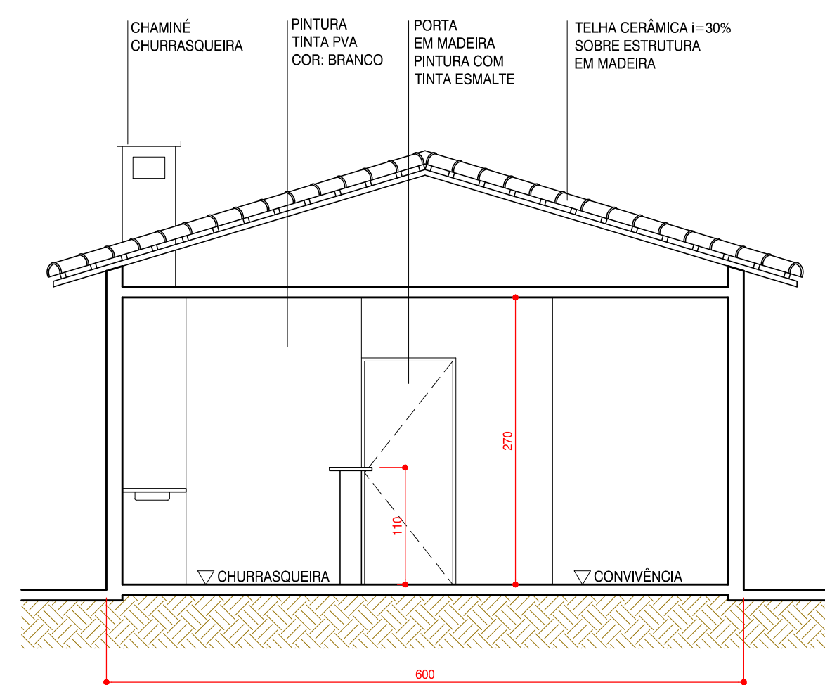
O3 CORTE 1:50
