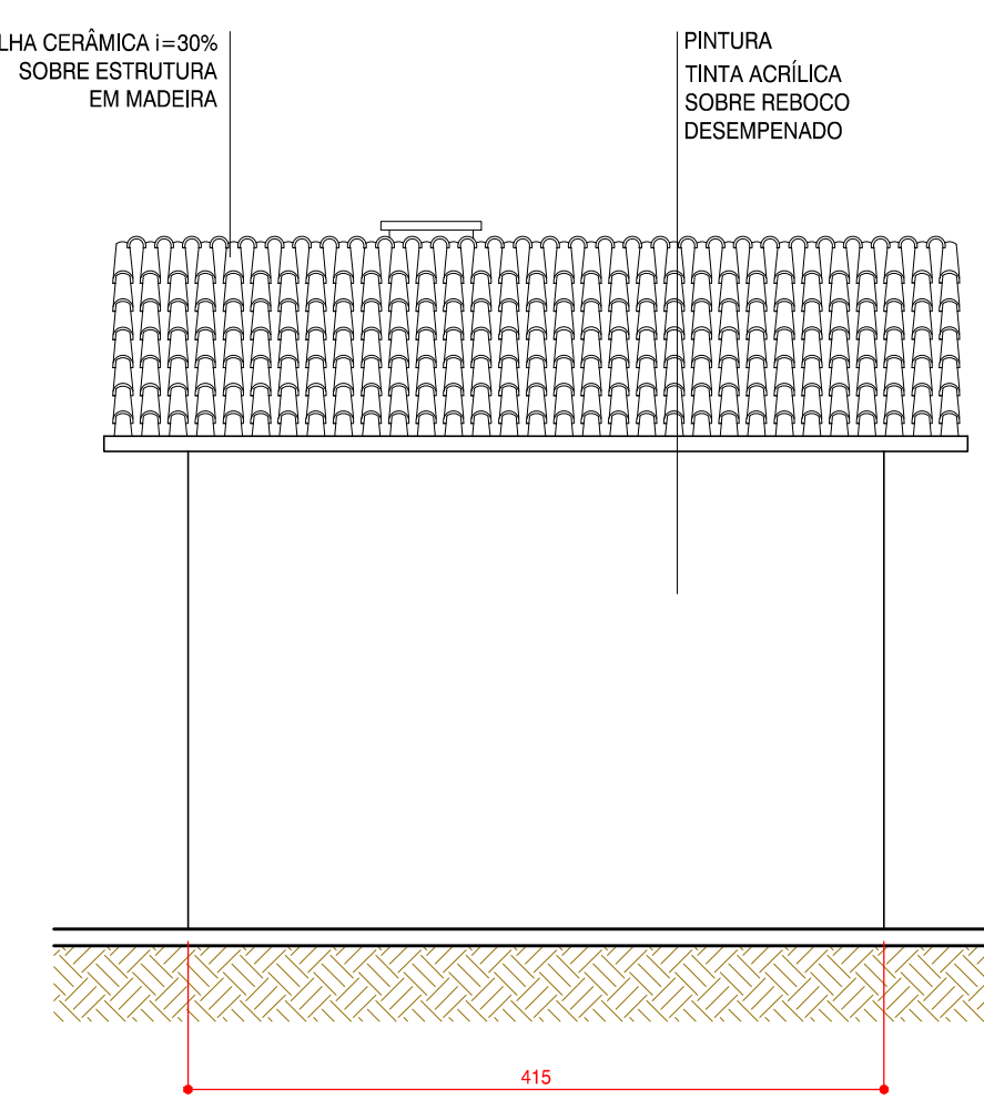
O9 ELEVACÃO 1:50
