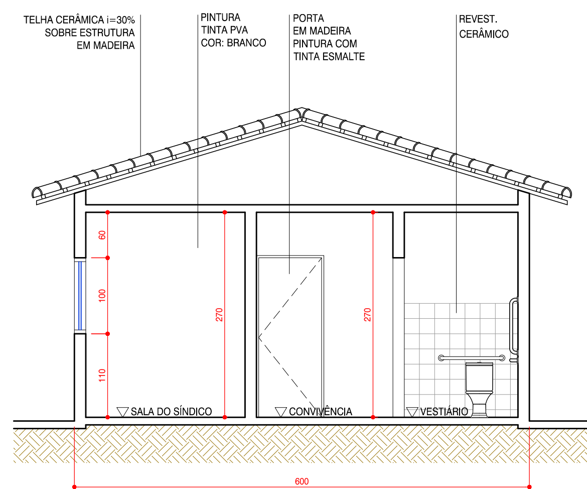
O4 CORTE 1:50
