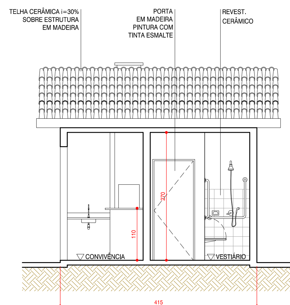
O5 CORTE 1:50
